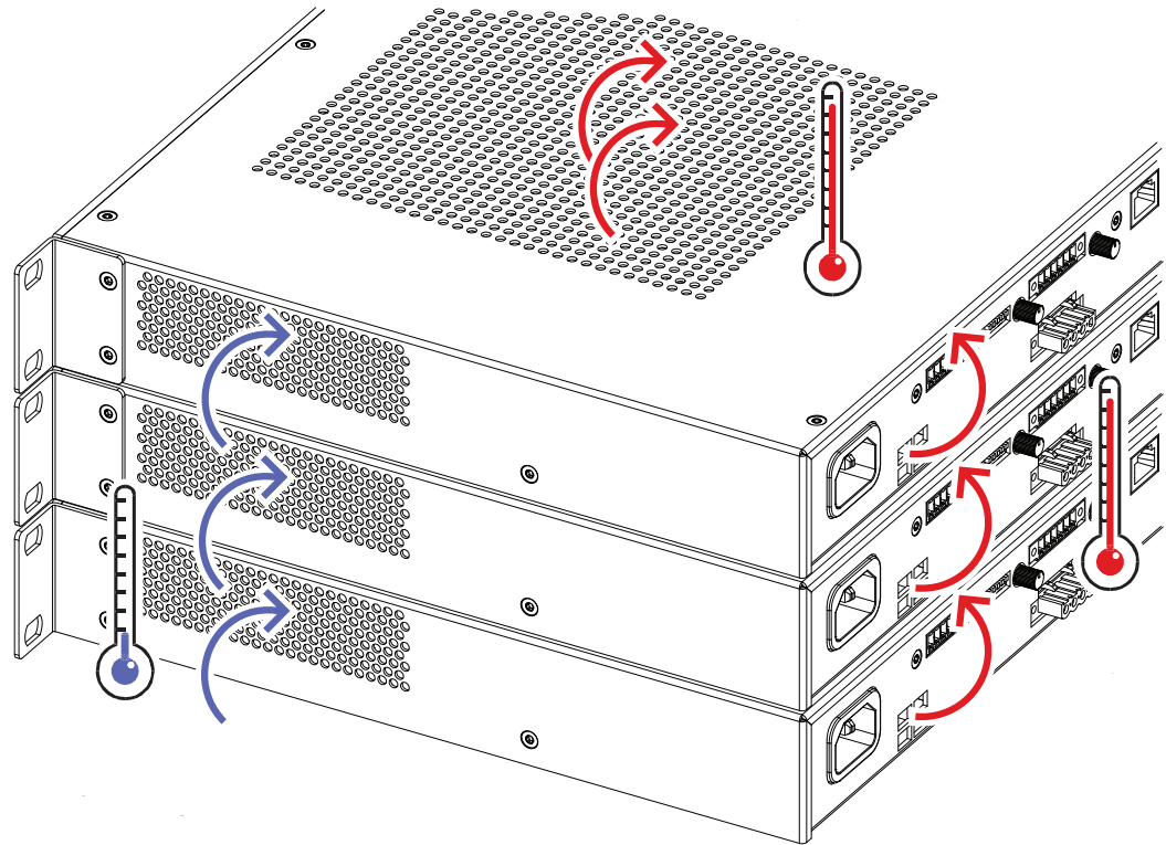
図 4.9: 複数の アンプのラックマウント。PRM-4P600 モデルの図。
