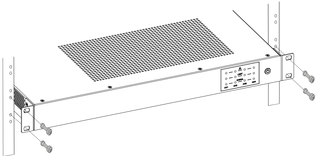
図 4.1: ラックへのアンプの取り付け
