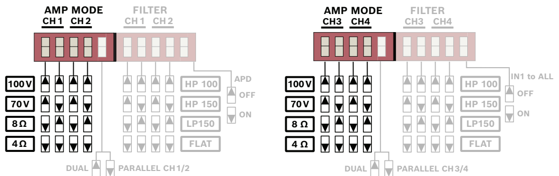
図 5.1: 出力モード設定 (PRM-4P600 のチャンネル 3 および 4 のみ)
