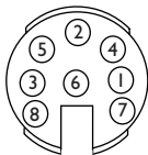
DC-diafragmaconnector 8-Pen connector (Gezien vanaf de solderzijde)
