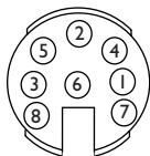
Conector de autoiris (Vista desde el lado del soldador)
