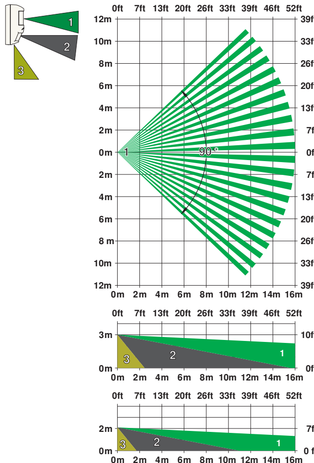
长距探测范围 16 米 x 21 米 (50 英尺 x 70 英尺)
