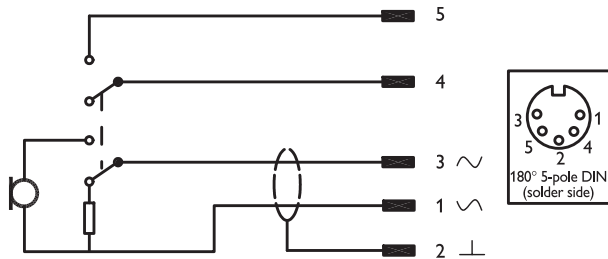
电路图
