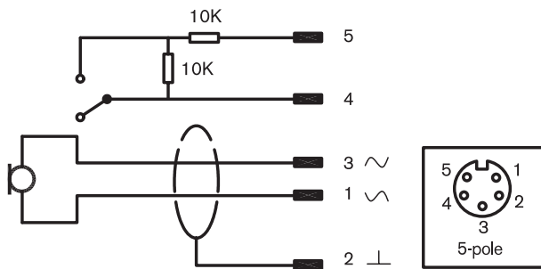
Kapcsolási rajz
