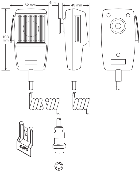
Méreték mm-ben
