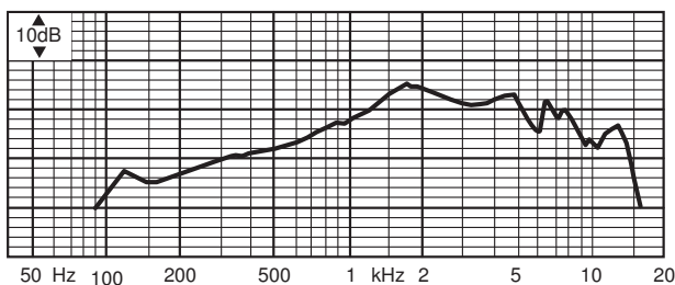
Απόκριση συχνότητας
