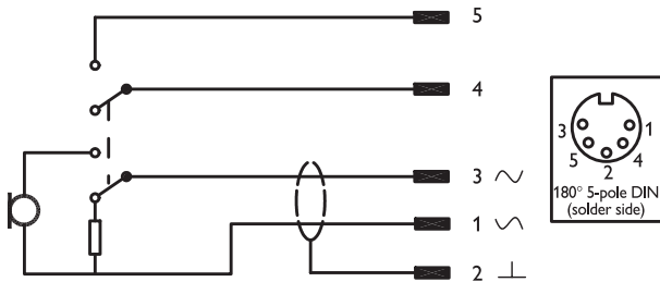
Διάγραμμα κυκλώματος
