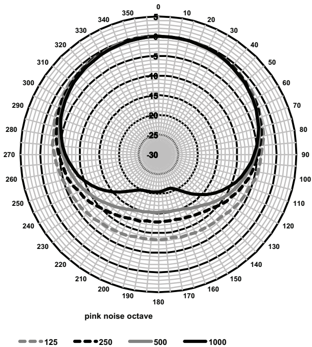
Afb. 2: Polair diagram (gemeten met roze ruis)
