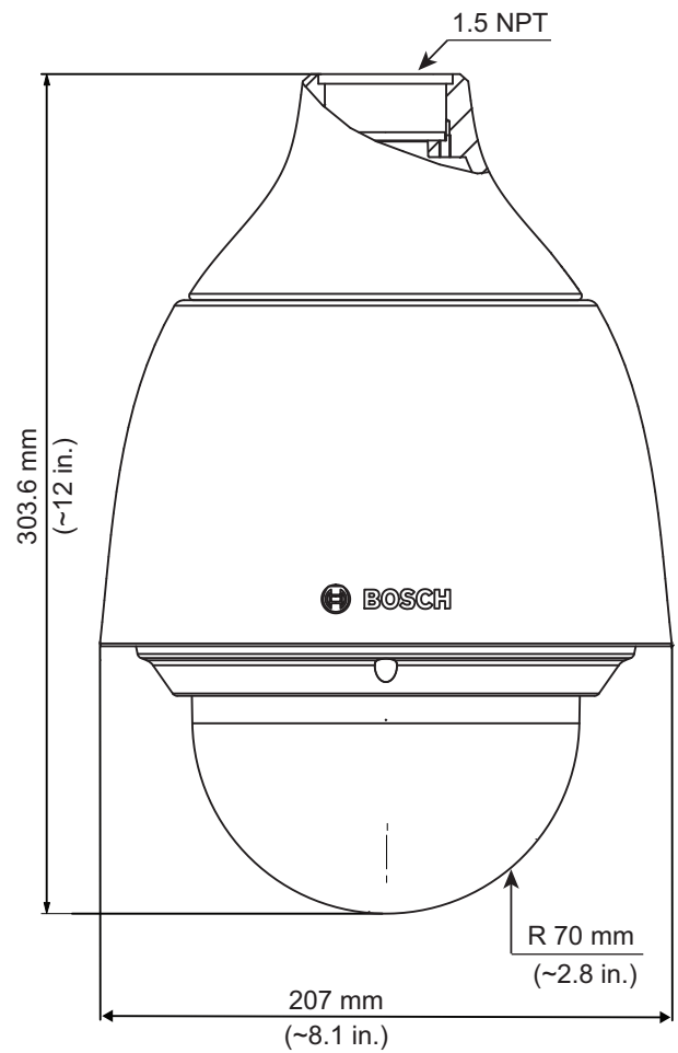
圖 7: 懸掛機型
