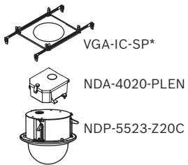
圖 5: 天花板掛架
