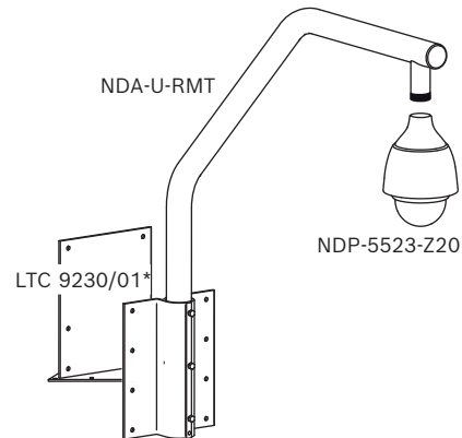
Afb. 4: Dakmontage (IP66)
