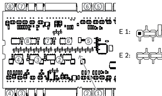
Rysunek 4.20: Umieszczenie zwór wyjść przekaźnikowych (spód płyty)
