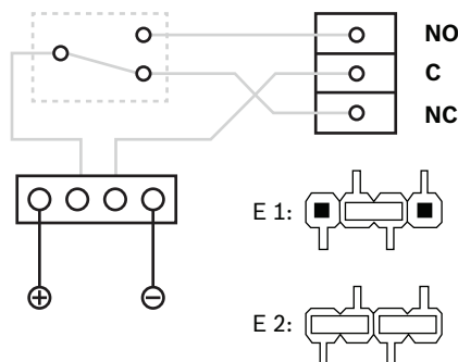
Rysunek 4.19: Ustawienia trybu przekaźnika
