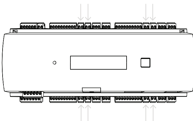
Rysunek 4.22: Umieszczenie złączy wejść analogowych
