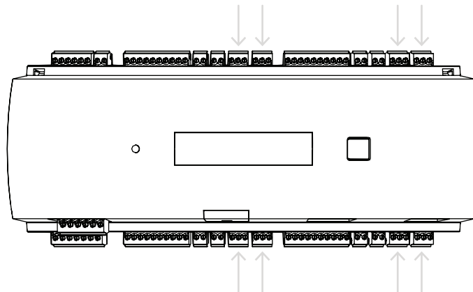
Rysunek 4.18: Umieszczenie złączy wyjść przekaźnikowych
