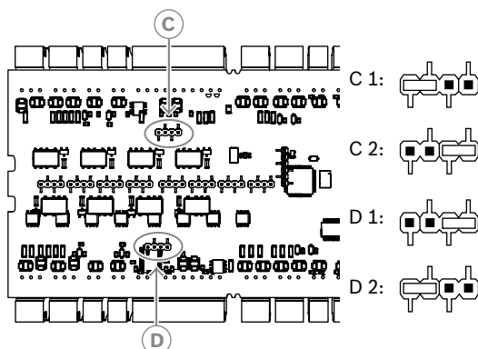
Rysunek 4.7: Położenie zwory masowej interfejsów magistrali
